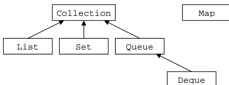
Einige Interfaces des Collections-Frameworks
